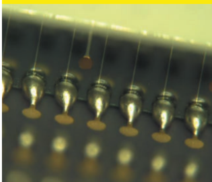
Вертикальный монтаж кристалла
